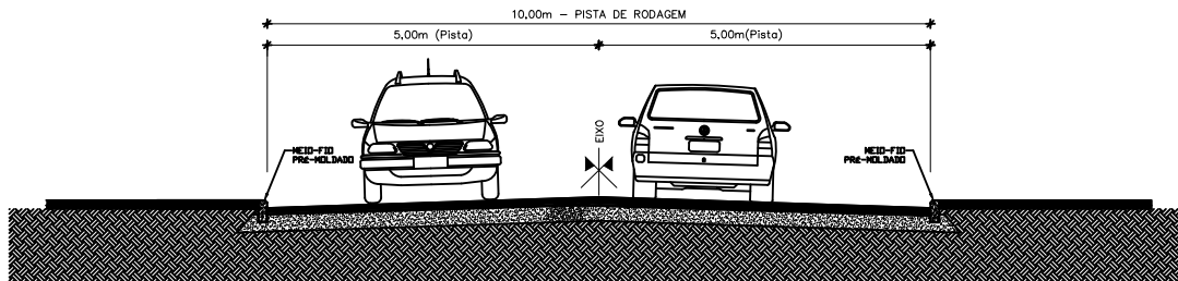
SEÇÃO TIPO DE PAVIMENTAÇÃO ASFÁLTICA - RUA MIRAGUAÍ
